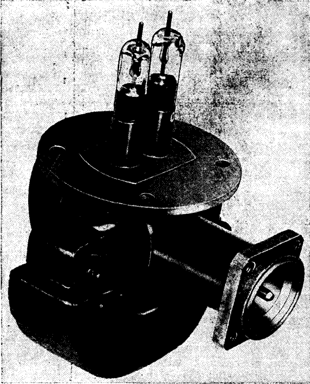
FIG. 19-15.—2J39 magnetron.
